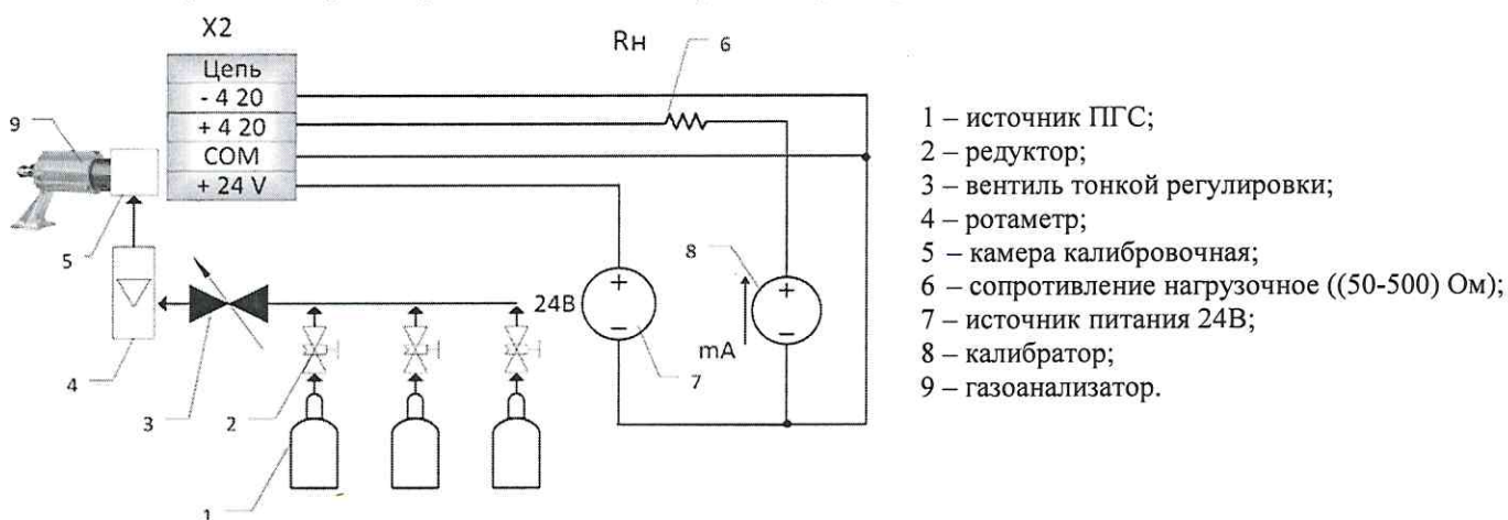
Рисунок 1 - Схема поверки газоанализатора
